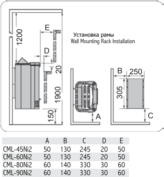
Рис. 1 | Минимальные безопасные расстояния (мм) Fig. 1 | Minimum safety distances (mm)
