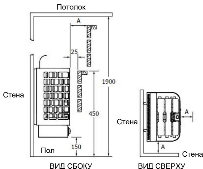
Рис. 1 Минимальные безопасные расстояния (мм)
