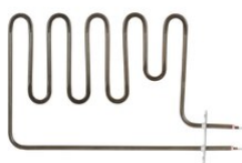
ТЭН SAWO HP65-004 (для электрических печей, Taurus, 1,0 кВт)
